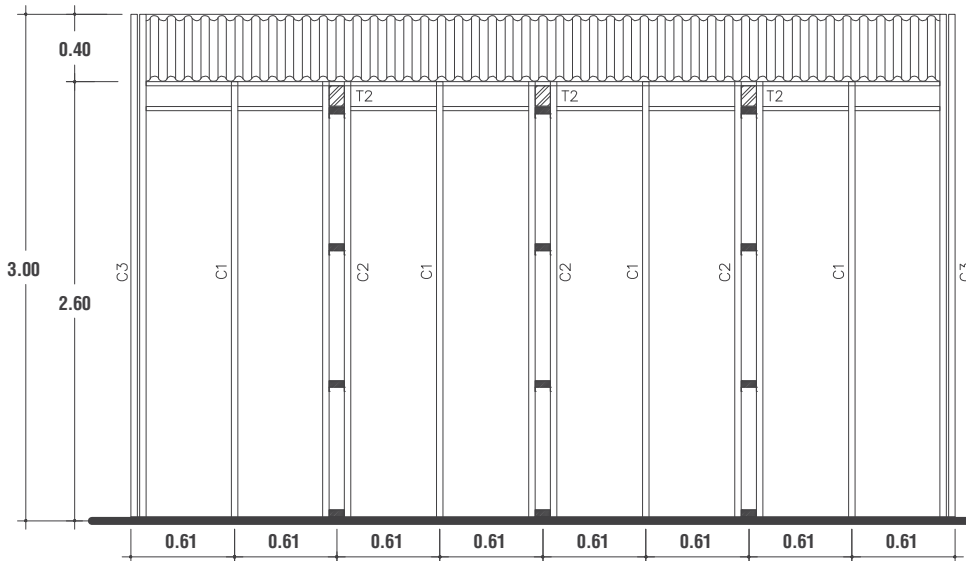
Elevación Posterior
