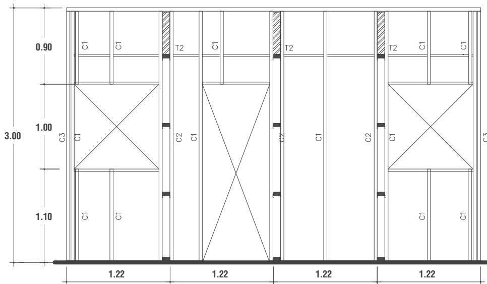
Elevación Frontal
